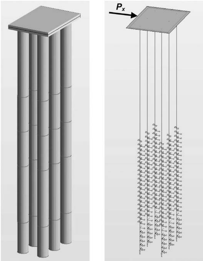
Rys. 3. Model geometryczny i schemat obliczeniowy dalby odbojowej
