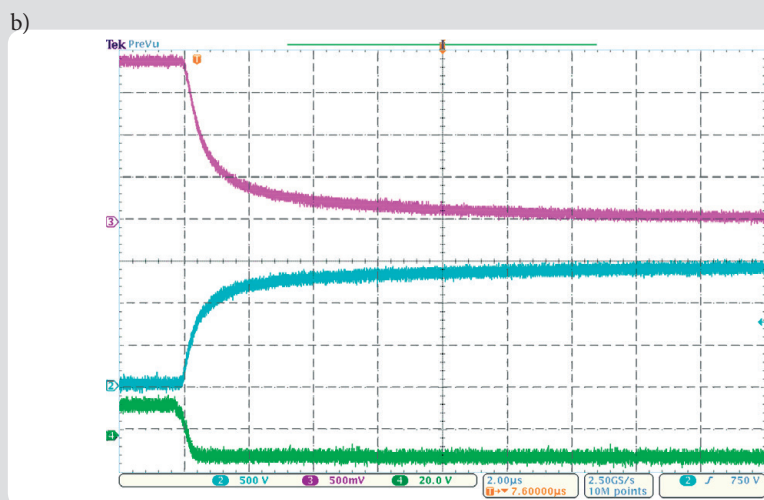
Rys. 4. Przebiegi uzyskane dla opracowanego półmostka IGBT w czasie załączania ( 1 \mu\text{s}/\text{dz} ) (a) oraz wyłączenia ( 2 \mu\text{s}/\text{dz} ) (b) wysokonapięciowego tranzystora IXLF19N250A. Od góry: prąd ( 2,5 \text{ A}/\text{dz} ), napięcie na tranzystorze ( 500 \text{ V}/\text{dz} ) oraz napięcie na bramce ( 20 \text{ V}/\text{dz} )
