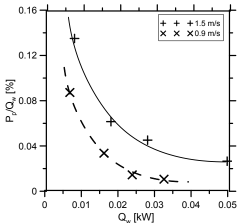
Rys. 8. Efektywność wymiany ciepła
