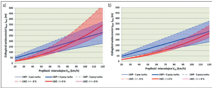
Rys. 2. Wykres zależności odległości widoczności na przejściu pieszym przez jezdnię L_{WP} i odległości widoczności na zatrzymaniu pojazdu przed przejściem L_{WZ} w zależności od prędkości miarodajnej V_{85} oraz wielkości pochylenia podłużnego jezdni na odcinku dojazdowym do przejścia dla pieszych w przypadku: a) normalnego hamowania, b) gwałtownego hamowania.
