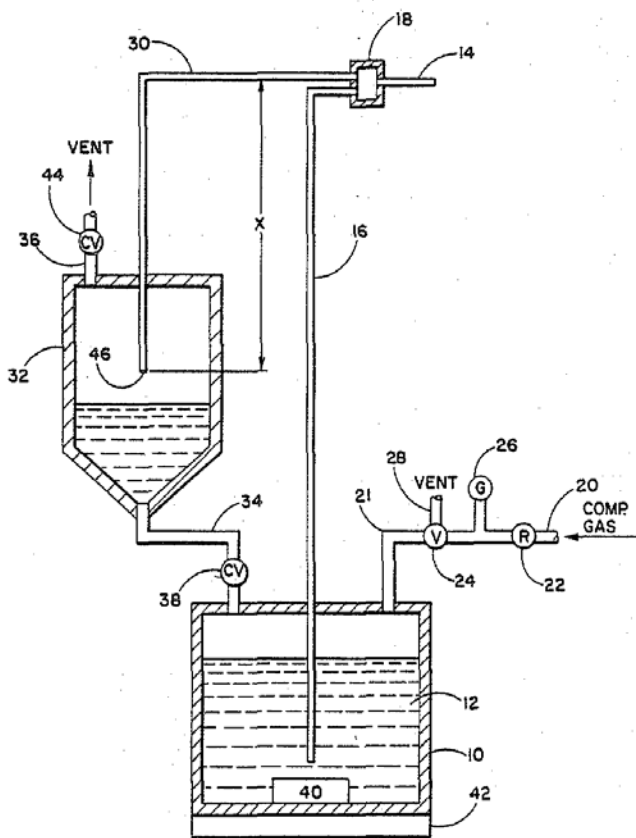
Rys. 4. Budowa układu dawującego zawiesinę ścierną z systemem oczyszczania dyszy i odzyskiem zawiesiny: 10 – zbiornik, 12 – zawieszona ścierna, 40 – mieszadło magnetyczne, 42 – magnes stały, 20 – przewód dostarczający powietrze, 22 – regulator ciśnienia, 26 – manometr, 24 – rozdzielacz trójdrogowy, 21, 28 – przewody, 16 – przewód dostarczający zawiesinę, 18 – komora, 14 – dysza rozpylająca zawiesinę ścierną, 30 – przewód sphywowy dla nadmiaru zawiesiny, 32 – zbiornik pośredni, 34, 38 – przewody, 38, 44 – zawory zwrotne [7]
