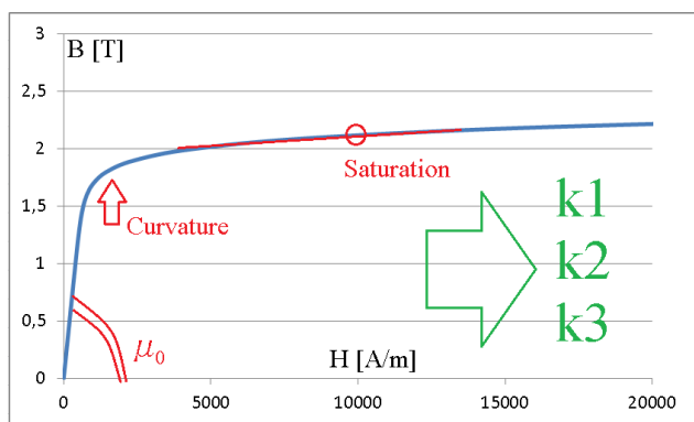
Rys. 4. Zmierzone lub pobrane z literatury parametry inżynierskie (przenikalność początkowa „ \mu_0 zero”, promień krzywizny „Curvature”, indukcja nasycenia „Saturation”) stanowią punkt wyjścia do wyznaczenia postaci analitycznej krzywej anhisterozowej B(H)
