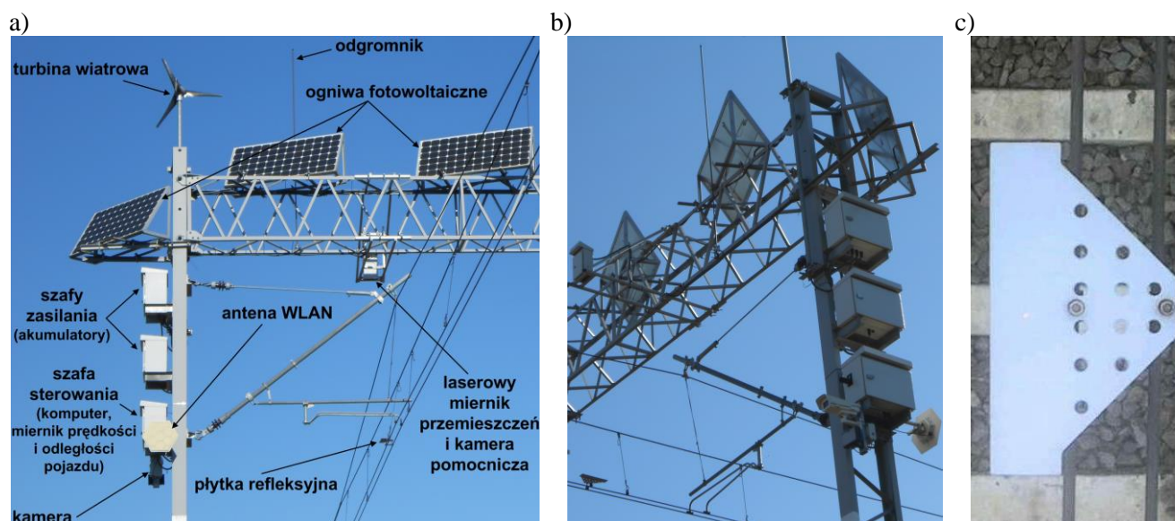
Rys. 3. Stanowisko pomiarowe: a) widok wzdłuż toru; b) widok z boku; c) płytkę refleksyjną
