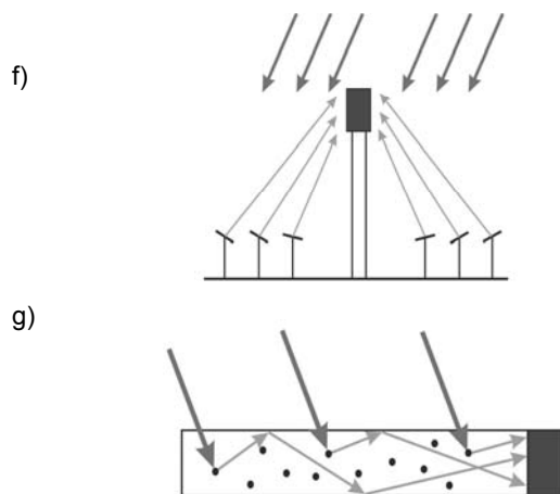
Rys. 1. Podstawowe metody koncentracji promieniowania słonecznego; a) klasyczna soczewka, b) soczewka Fresnela, c) zwierciadło paraboliczne, d) zwierciadło wklęsłe-liniowe, e) liniowa soczewka Fresnela, f) system zwierciadeł skupiających promieniowanie na wieży oraz g) koncentratory luminescencyjne (na podstawie [2])
