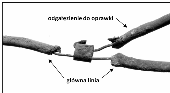
Rys. 12. Sposób łączenia kabli wewnątrz złączki
