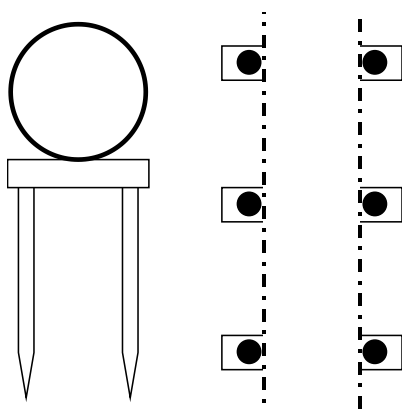
Rys. 2. Przykład nieprawidłowego posadowienie rurociągu w podłożu gruntowym
