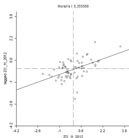
Rysunek 6. Wykres Morana dla zmiennej zgonów w przekroju podregionów
