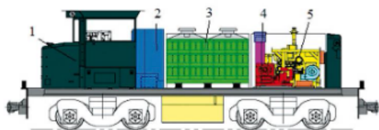
Rys. 3. Układ napędowy lokomotywy GK10B Railpower Technologies Corp. [13 ]: 1 - kabina maszynisty, 2 - wyposażenie elektryczne, 3 - moduł baterii, 4 - sprężarka powietrza, 5 - zespół napędowy (silnik-prądnica)
