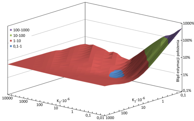
Rys.6. Wykres błędu odtwarzania położenia kąowego na wyjściu obserwatora ATO w funkcji wzmoceń K_1 i K_2
