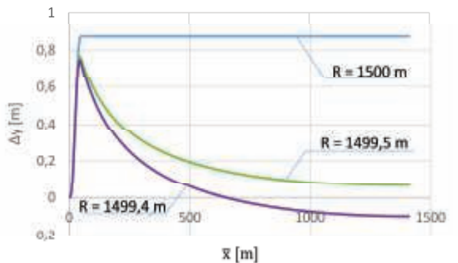
11. Wykresy różnic rzędnych na długości zmodyfikowanego układu geometrycznego dla R = 1500\text{ m} , 1499,5\text{ m} i 1499,4\text{ m} , l_k = 70\text{ m} , l_w = 130\text{ m} ( \alpha = 135^\circ )
