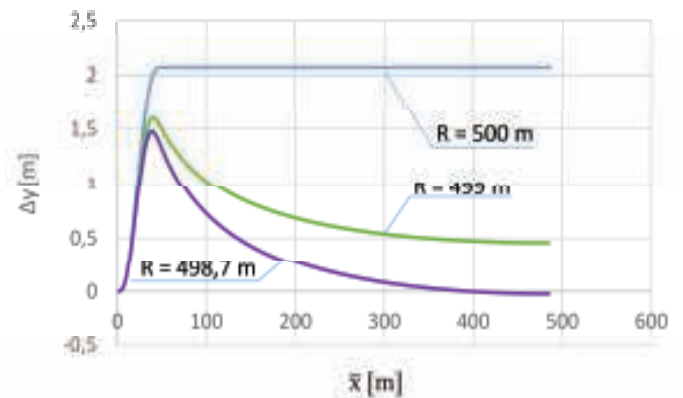
9. Wykresy różnic rzędnych na długości zmodyfikowanego układu geometrycznego dla R = 500\text{ m} , 499\text{ m} i 498,7\text{ m} , l_k = 70\text{ m} , l_w = 120\text{ m} ( \alpha = 135^\circ )
