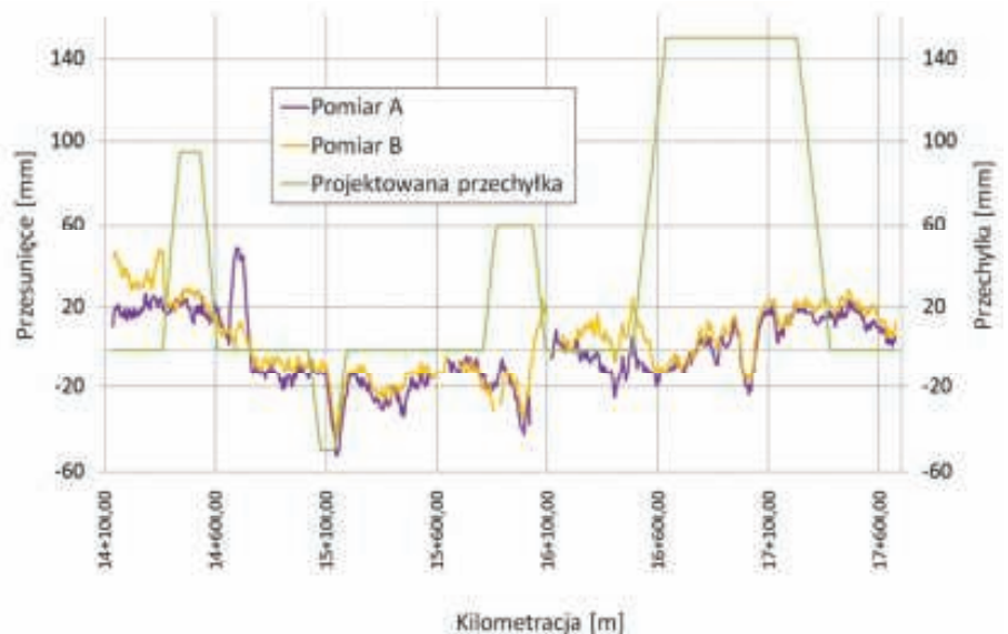
6. Wykresy przesunięć dla toru nr 2
