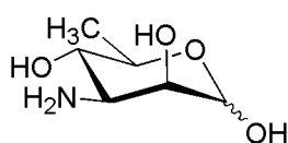
D-mycosamine
