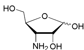
D-ribosamine
