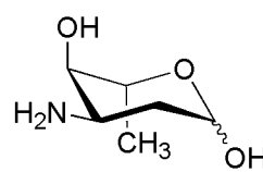
L-ristosamine
