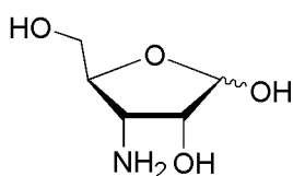
D-ribosamine
