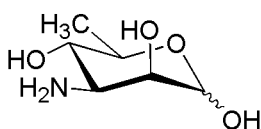
D-mycosamine
