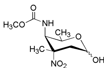
D-kijanose
