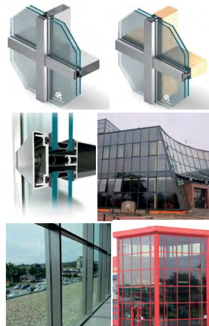
Rys. 4. Przykłady rozwiązań konstrukcyjnych ścian słupowo-ryglowych
