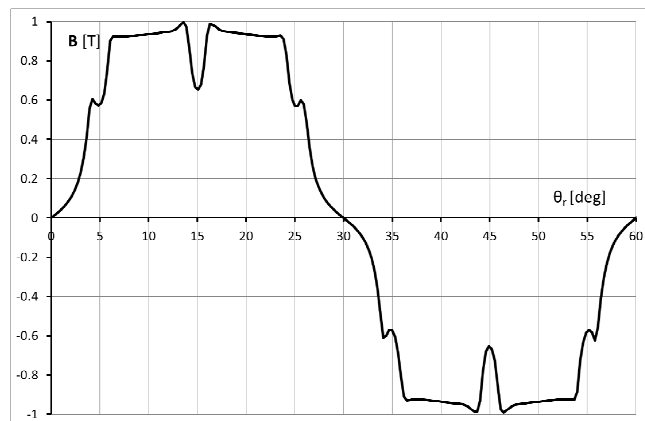
Rys. 4. Rozkład składowej normalnej wektora indukcji magnetycznej w szczelinie roboczej GMT
