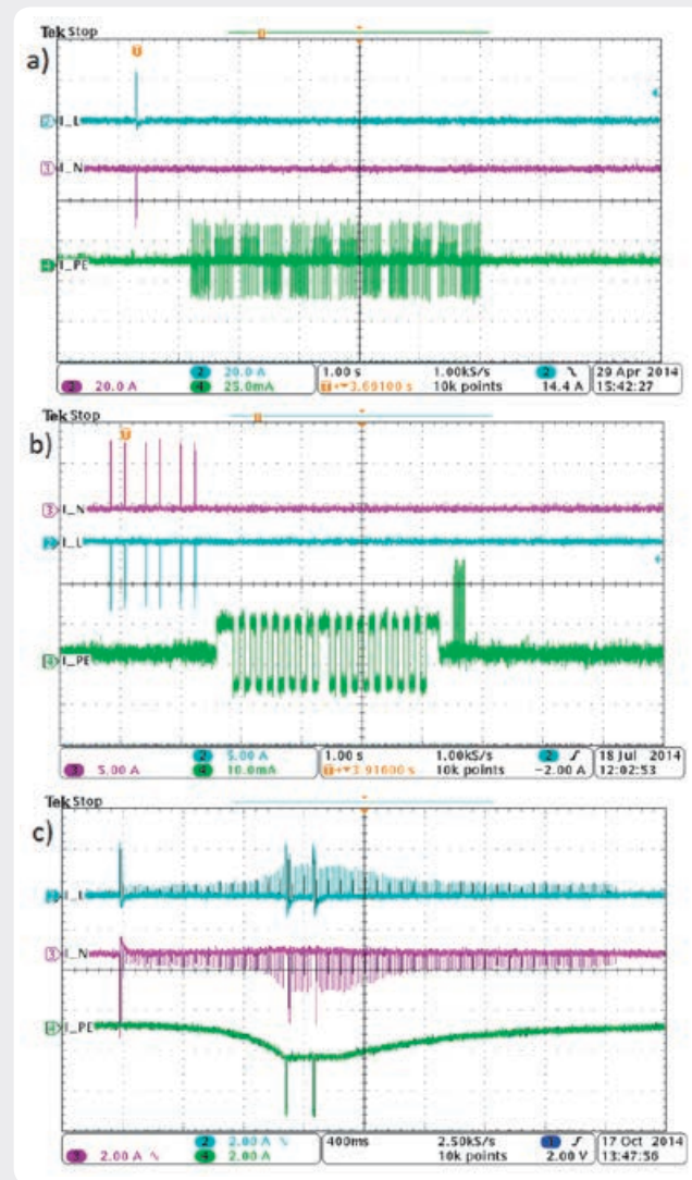
Rys. 5. Przebiegi prądów w przewodach L, N i PE podczas pomiaru z aktywną funkcją ATT/RCD, a) Sonel MPI-520 (skala: I_L, I_N - 20 \text{ A/dz.} , I_{PE} - 25 \text{ mA/dz.} ), b) Kyoritsu KEW 4140 (skala I_L, I_N - 5 \text{ A/dz.} , I_{PE} - 10 \text{ mA/dz.} ), c) Kyoritsu 4120A (skala 2A/dz.)
