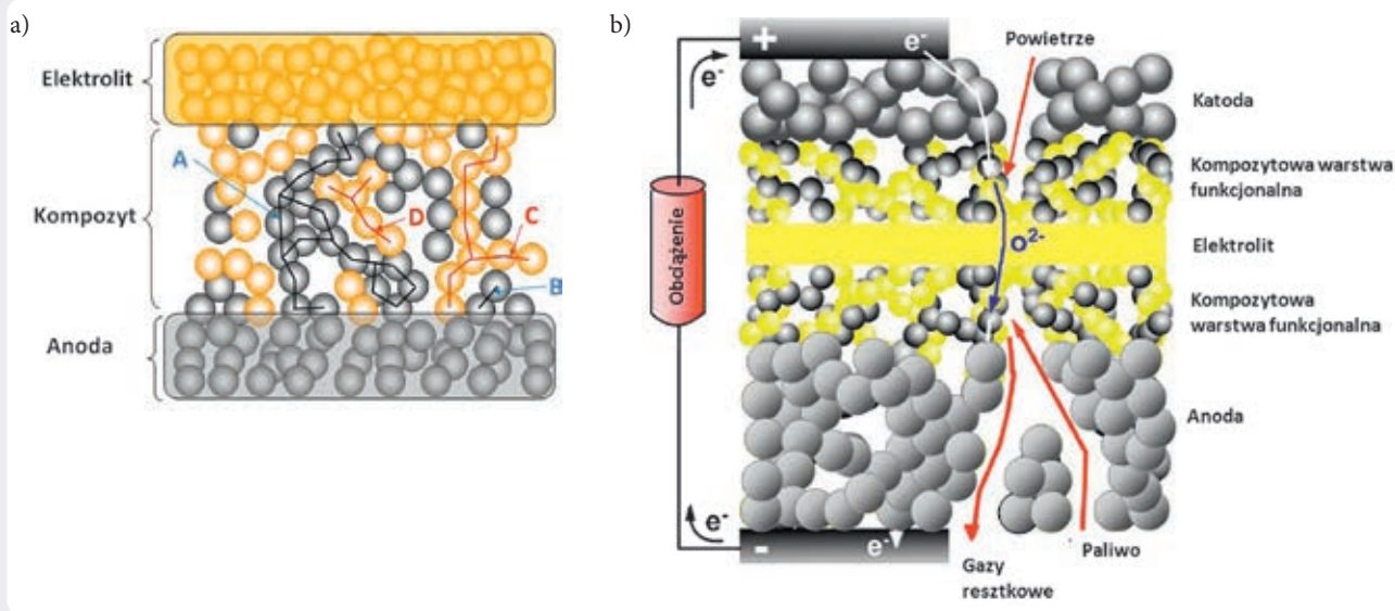
Rys. 2. Schemat idealowy układu warstw w ogniwie SOFC.
