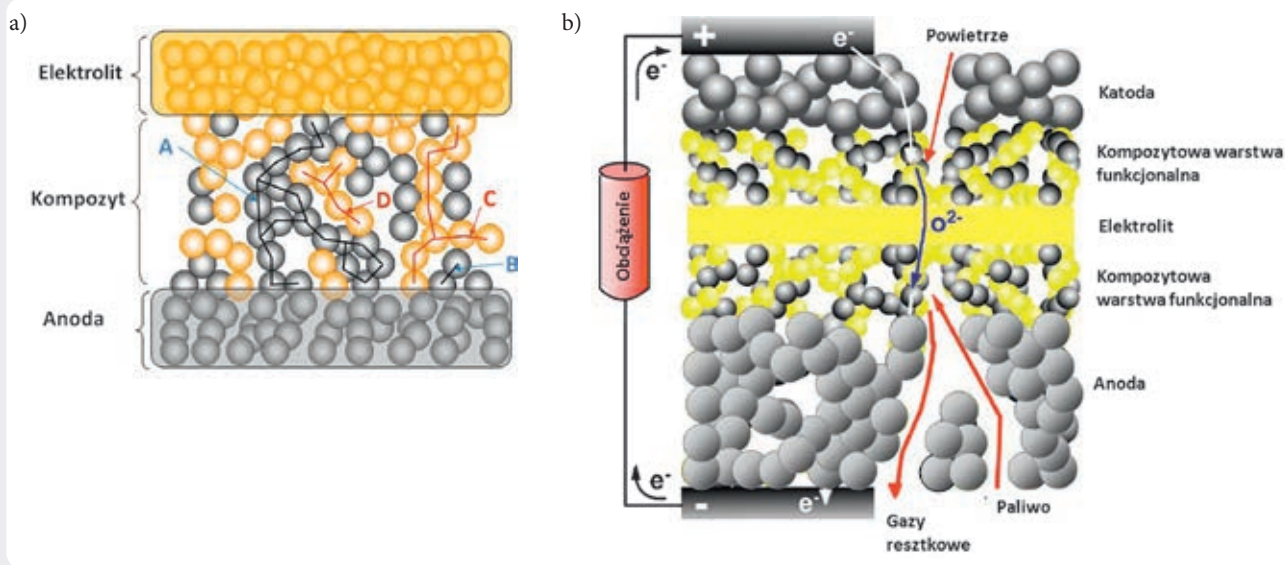
Rys. 2. Schemat ideowy układu warstw w ogniwie SOFC.
