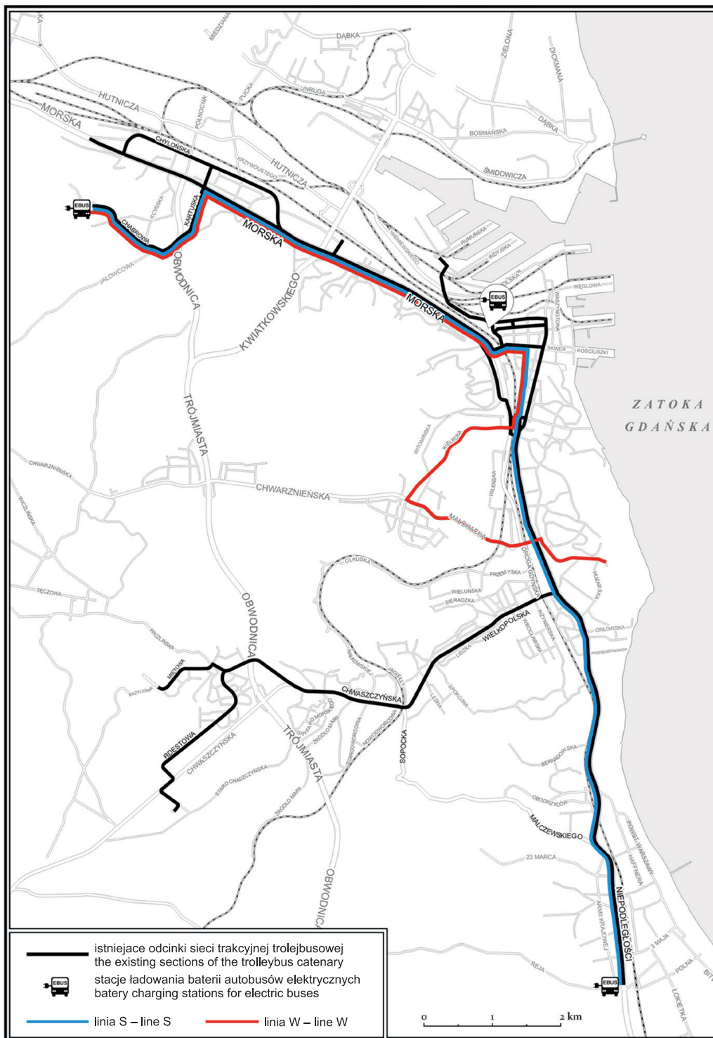
Rys. 2. Schemat linii autobusowych wyznaczonych jako potencjalne do obsługi autobusami elektrycznymi (elektrobusami)
