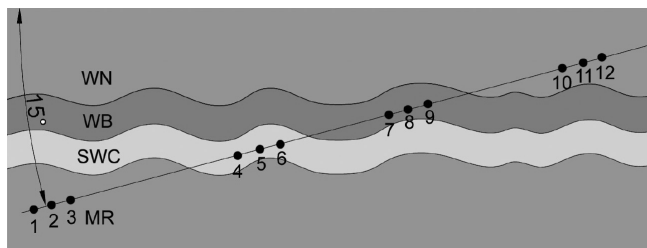
Rys. 4. Schemat pomiaru twardości w próbce napawanej: MR – materiał rodzimym, SWC – strefa wpływu ciepła, WB – warstwa buforowa napawana spoiwem 309LMo, WN – warstwy napawane spoiwem 316L
