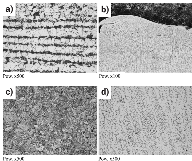
Rys. 3. Mikrostruktury poszczególnych obszarów próbki napawanej: a) materiał rodzimym, b) strefa: napoina – linia wtopienia, c) SWC, d) napoina. Trawienie stali niestopowej Nital / napoina \text{HCl}/\text{C}_6\text{H}_3\text{N}_3\text{O}_7/\text{C}_2\text{H}_5\text{OH}
