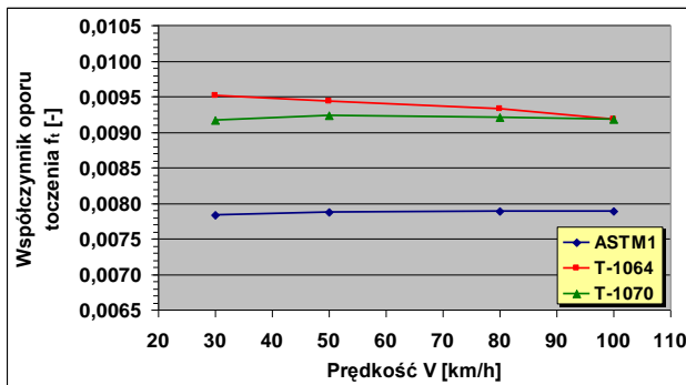
Rys. 1. Zależność oporu toczenia opony od prędkości na nawierzchni DAC dla trzech opon
