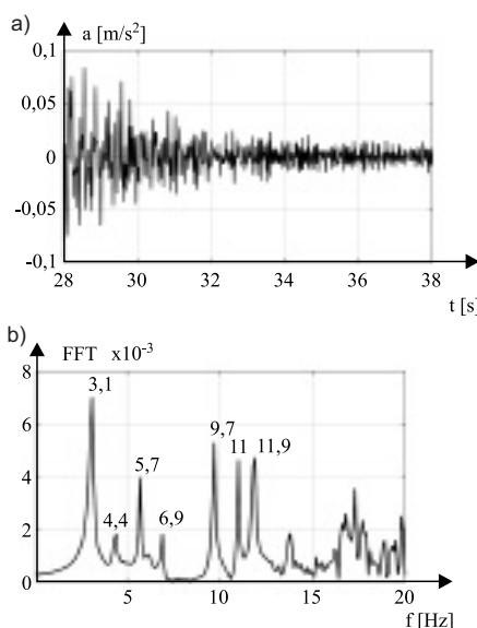
Rys. 2. Swobodna odpowiedź kładki [1]: a) zarejestrowana składowa pionowa przyspieszeń b) analiza FFT
