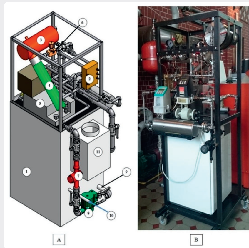
Rys. 2. Mikrośiwnia ORC; (A) rysunek aksjonometryczny: 1 – kocioł gazowy, 2 – parownik, 3 – turbogenerator, 4 – skraplacz, 5 – zbiornik etanolu, 6 – zawór dławiący, 7 – przepływomierz oleju, 8 – pompa oleju, 9 – króciec powrotu oleju do kotła, 10 – króciec gazowy, 11 – czopuch; (B): widok stanowiska
