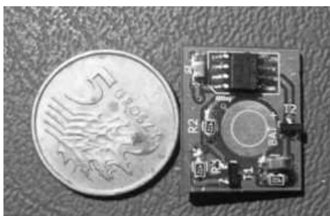
Rys. 4. Zrealizowany moduł zasilający na bazie przetwornicy MAX1796 (bez diody świecącej)
