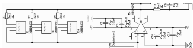
Rys. 4. Fragment głowicy pomiarowej z przedwzmacniaczem
