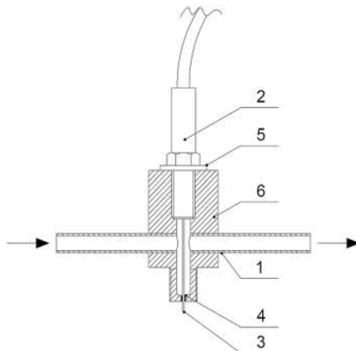
Rys. 4. Przekrój poprzeczny termopary typu K umieszczonej w płaszczu wodnym: 1 – króćce zasilające i odprowadzające wodę chłodzącą, 2 – chłodzona termopara ze spiną zgrzewaną do płaszcza, 3 – spina pomiarowa, 4 – izolacja termiczna płaszcza termopary, 5 – uszczelka, 6 – osłona termopary
