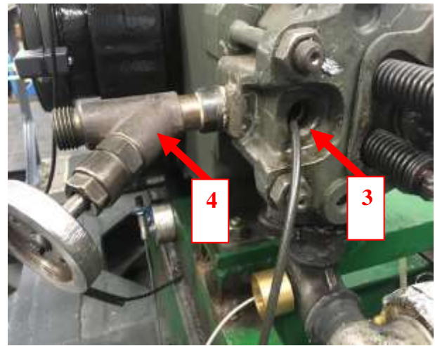
Rys. 4. Widok ogólny stanowiska laboratoryjnego silnika Farymann Diesel typu D10 przygotowanego do badań endoskopowych (a), sposób wprowadzenia sondy inspekcyjnej wideoendoskopu do przestrzeni roboczej silnika (b): 1 – silnik Farymann Diesel typu D10; 2 - wideoendoskop pomiarowy Everest typu XLG3 przygotowany do badania silnika; 3 – otwór wziernikowy po zdemontowanym wtryskiwaczu; 4 – zawór indykatorowy
