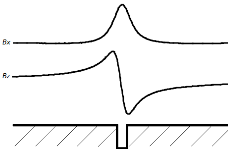
Rys. 2.5. Rozkład przestrzenny dwóch składowych indukcji MPR - równoległej B_x i normalnej B_z do powierzchni próbki - nad ubytkiem materiału o długości 2 mm i głębokości 8 mm
