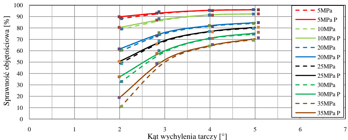
Rys. 9.36 Sprawność objętościowa w funkcji kąta wychylenia tarczy dla różnych \Delta p dla v=120cSt i n=500obr/min . P – oś obrotu przesunięta o h=D/2
