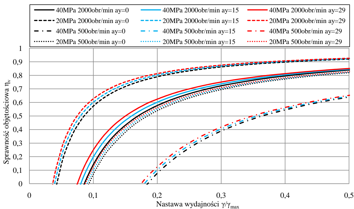
Rys. 8.20 Symulacja przebiegu sprawności objętościowej dla pompy Parker PV023; \alpha_s=0 ; K=1700\text{MPa} ; D=58\text{mm} ; d_t=14,15\text{mm} ; \gamma_{\max}=15,65^\circ ; V_{\text{min}}=4275\text{mm}^3 ; \nu=40\text{cSt} ; h_r=10\mu\text{m} ; h_s=10\mu\text{m} ; \alpha=0,017^\circ
