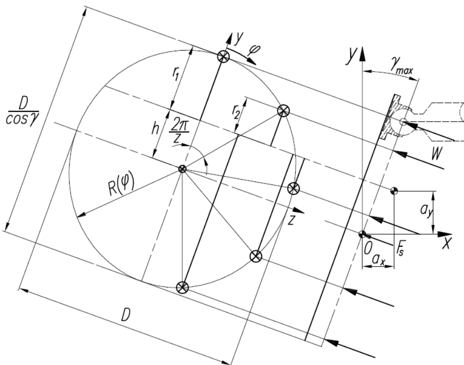
Rys. 8.21 Obciążenie wychylnej tarczy i zmiana momentów od poszczególnych tłoczków w fazie tłoczenia przy przeszczaniu osi obrotu tarczy o a_x i a_y wyznaczonymi dla \gamma_{max}
