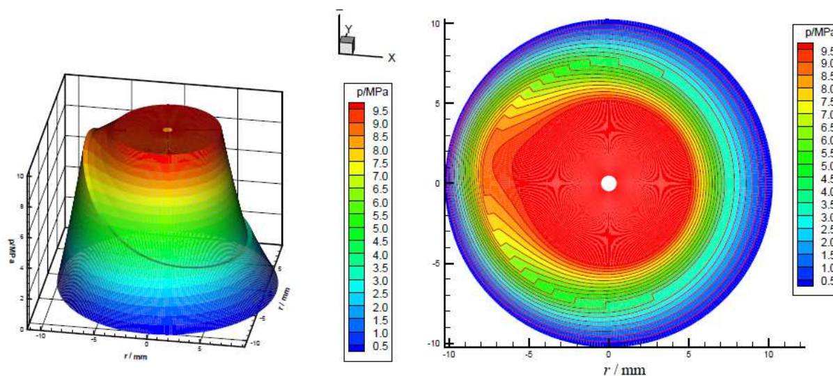
Rys. 1.14 Wyniki analizy CFD rozkładu pola ciśnień pod stopką. Ciśnienie w komorze cylindrowej p=10\text{MPa} , kąt nachylenia stopki \alpha=0,05^\circ , prędkość obrotowa \omega=25,12\text{ rad/s} [10]
