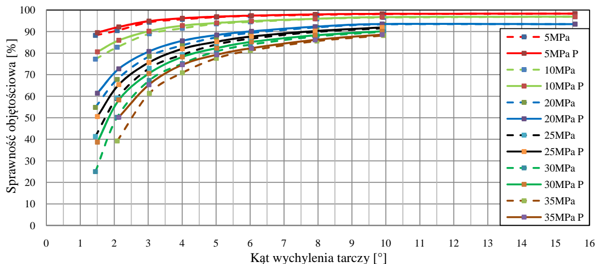
Rys. 9.35 Sprawność objętościowa w funkcji kąta wychylenia tarczy dla różnych \Delta p dla v=80cSt i n=2000obr/min . P – oś obrotu przesunięta o h=D/2
