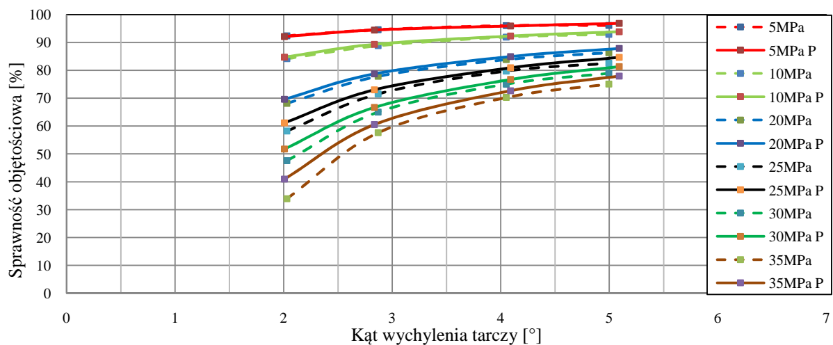
Rys. 9.37 Sprawność objętościowa w funkcji kąta wychylenia tarczy dla różnych \Delta p dla v=120cSt i n=1000obr/min . P – oś obrotu przesunięta o h=D/2
