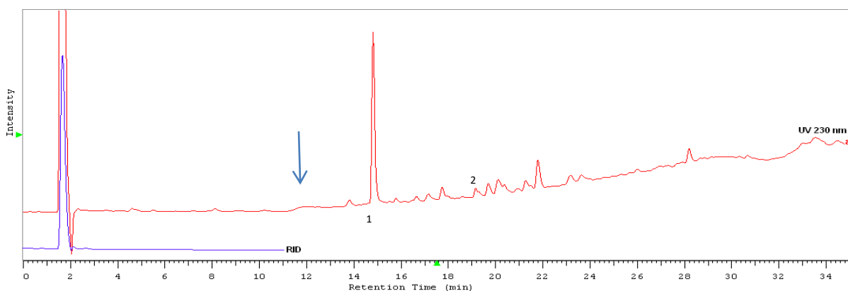
Rys. 38. Nałożone chromatogramy z detektora RID (niebieska linia) oraz UV 230 nm (czerwona linia) -5% \text{Na}_2\text{CO}_3 Hydrolyzate , temp. 90°C, czas: 24 h — objętość dozowana - 50 \mu\text{l} , warunki rozdzielania: metoda B , Piki: 1- kwas 4-hydroksybenzoesowy, 2- kwas 3,4-dihydroksybenzoesowy, reszta pików niezidentyfikowana-powiększenie
