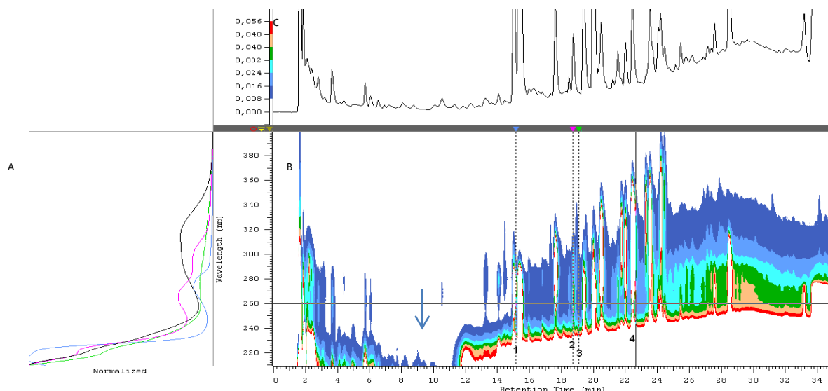
Rys. 21. Chromatogram rozdzielania hydrolizatu wierzby energetycznej, warunki hydrolizy: katalizator: 5% \text{Ca(OH)}_2 , temp. 90°C, czas: 24 h, warunki rozdzielania: metoda B, objętość dozowana: 50 \mu\text{l} , A –widma wybranych składników, B – Chromatogram detektora UV-VIS DAD w odwzorowaniu poziomym, C-Chromatogram dla 260 nm, Piki: 1- kwas 4-hydroksybenzoesowy, 2- kwas 3,4-dihydroksybenzoesowy, 3- kwas 4-OH-3,5-metoksybenzoesowy i 4-hydroksy-3-metoksybenzaldehyd, 4- kwas t-ferulowy, reszta pików niezidentyfikowana
