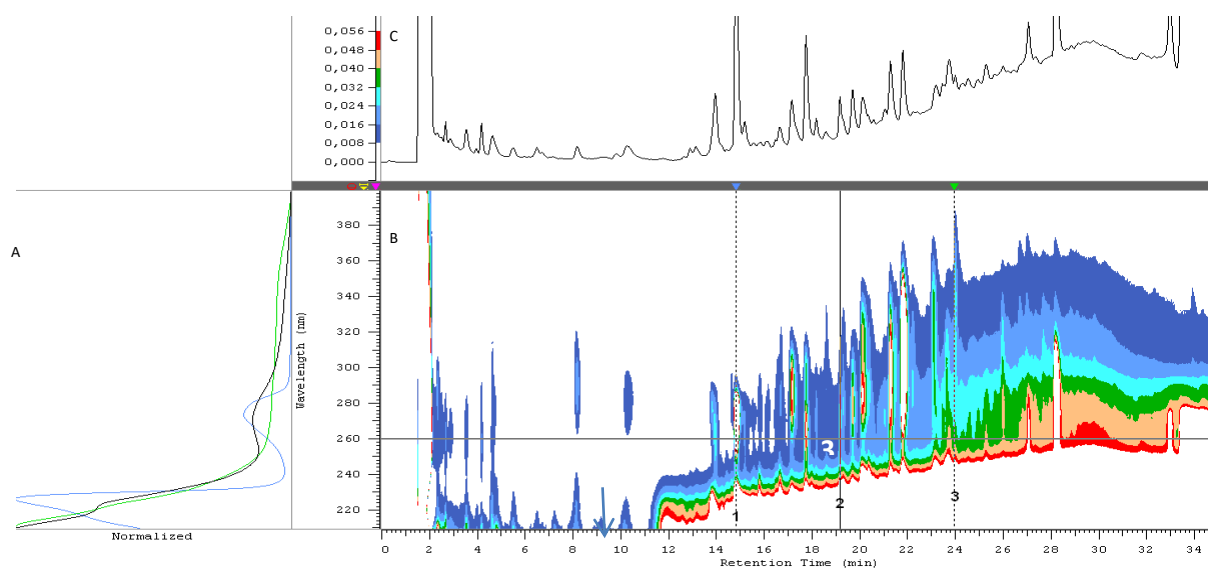
Rys. 22. Chromatogram rozdzielania hydrolizatu wierzby energetycznej, warunki hydrolizy: katalizator: 5% \text{Na}_2\text{CO}_3 , temp. 90°C, czas: 24 h, warunki rozdzielania: metoda A, objętość dozowana: 50 \mu\text{l} , A –widma wybranych składników, B – Chromatogram detektora UV-VIS DAD w odwzorowaniu poziomym, C-Chromatogram dla 260 nm, Piki: 1- kwas 4-hydroksybenzoesowy, 2- kwas 3,4-dihydroksybenzoesowy, 3-2,6-dimetoksyfenol, reszta pików niezidentyfikowana
