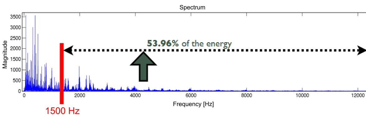
Fig. 3. Brightness (MIRtoolbox).
