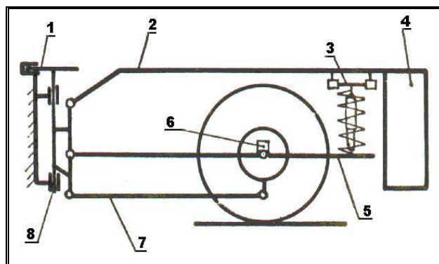
Rys. 2. Schemat kinematyczny przyczepy [3]: 1 – hamulec sworznia przyczepy, 2 – wahacz obciążników, 3 – przetwornik siły pionowej, 4 – obciążniki, 5 – wahacz badanego koła, 6 – przetwornik przyśpieszeń, 7 – ciągnio jarzma hamulca badanego koła, 8 – sworzień pionowy przyczepy.
