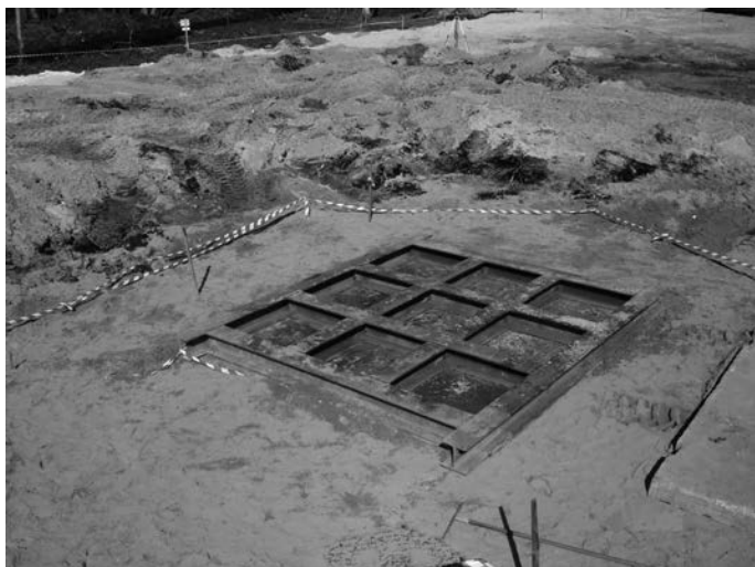
Rys. 5. Podstawa konstrukcji obciążającej kolumnę z kruszywa
