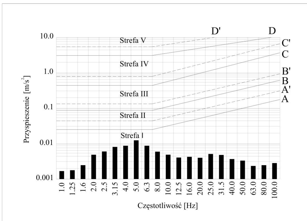
Rys. 3.22. Wyniki analizy dla budynku nr 7, wykonanej dla przejazdu samochodu osobowego do 3,5 t, naniesione na SWD II.
