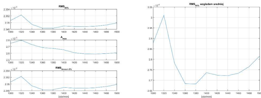
Rys 4. Wartości wskaźników poziomu drgań uzyskane w wyniku symulacji procesu skrawania, procedura modalna, powierzchnia 1
