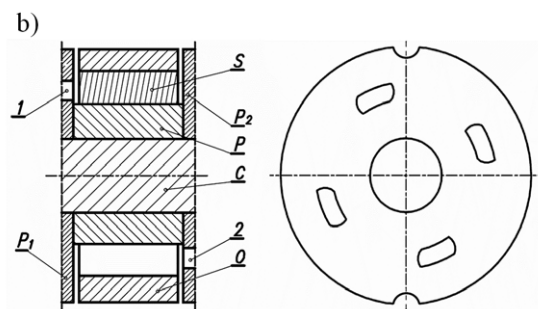
Rys. 6. Pompa z wirującą obwodnicą: a) kształt zarysu: O – obwodnica; P – planeta, S – satelity; b) luzy w mechanizmie i kształt płyty rozrzędu [5, 6]
