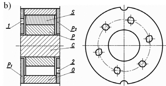
Rys. 5. Pompa z wirującą planetą: a) kształt zarysu: O – obwodnica, P – planeta, S – satelity; b) luzy w mechanizmie i kształt płyty rozrzędu [3]
