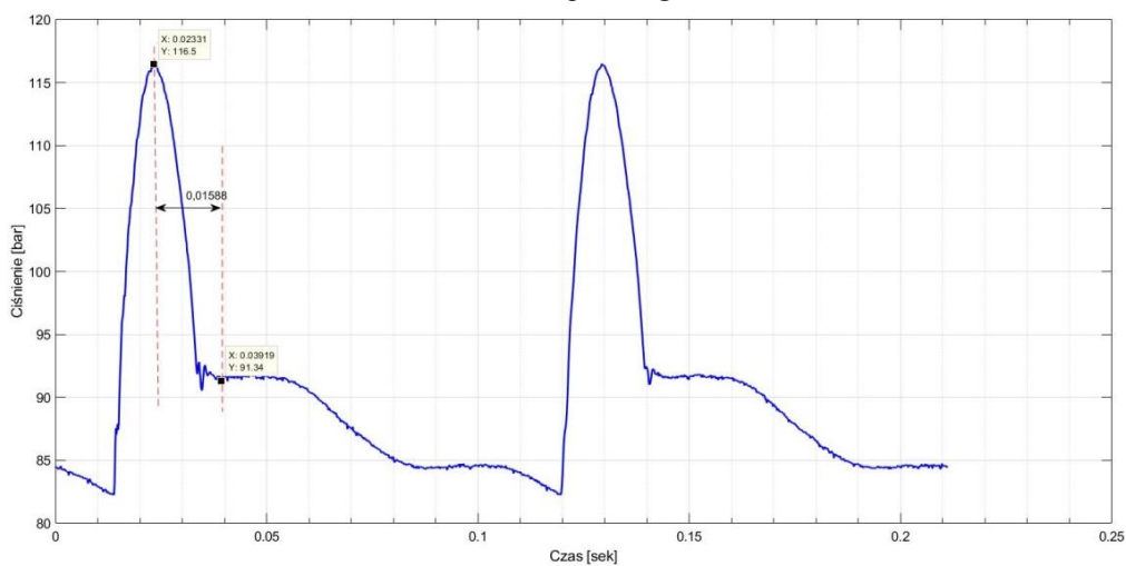
Rys. 4.4. Przebieg ciśnienia paliwa w przewodzie wtryskowym jako funkcji czasu z naniezionymi wartościami wielkości charakterystycznych
