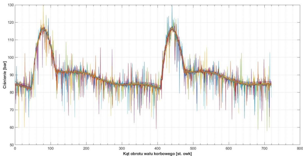
Rys. 4.2. Zarejestrowany sygnał ciśnienia w przewodzie wtryskowym – sygnał „zaszumiony”, naniezione około 500 przebiegów ciśnienia
