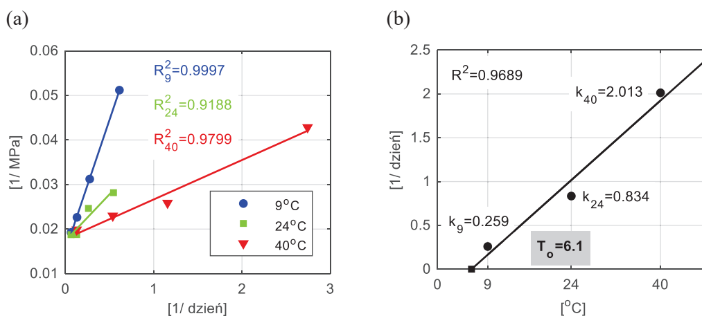
Rys. 4.14. Procedura zmodyfikowana ( \text{proc1\_v2} ): (a) odwrotność wytrzymałości w funkcji odwrotności wieku pomniejszonego o koniec wiązania, (b) zależność stałych k od temperatury pielęgnacji
