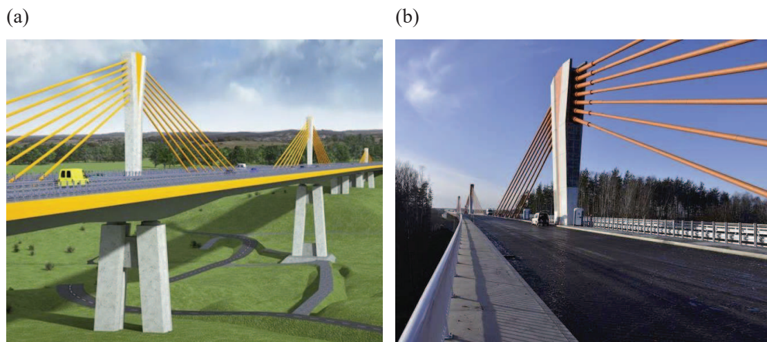
Rys. 5.2. (a) Wizualizacja obiektu MS-3B [171], (b) Widok wykonanego mostu extradosed [165]
