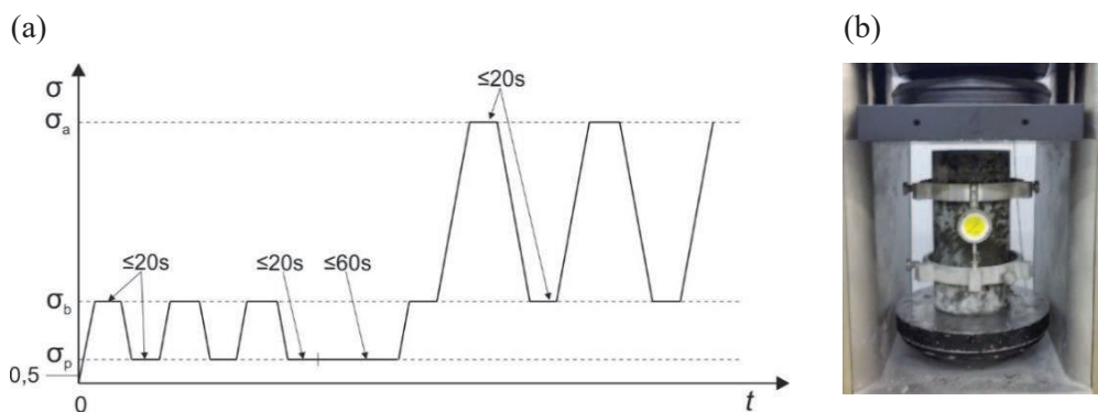
Rys. 4.42. (a) Schemat obciążenia cyklicznego w metodzie A [151], (b) Próbką z zamontowanym modułowierzem do pomiaru odkształceń betonu
