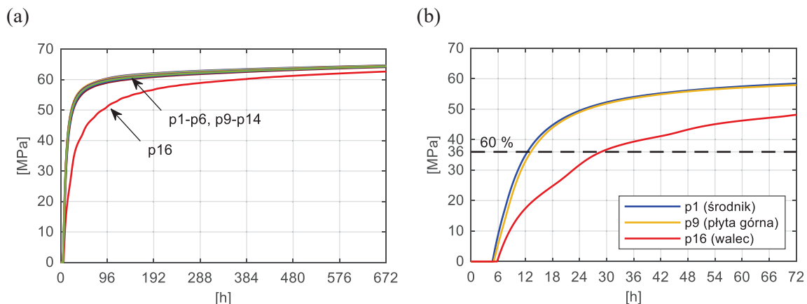
Rys. 5.39. Wytrzymałość walcowa betonu środника i płyty górnej (wg p1 - p6, p9 - p14) oraz próbki walcowej (wg p16) w funkcji czasu: (a) 672 h=28 dni, (b) 72 h (wybrane punkty)
