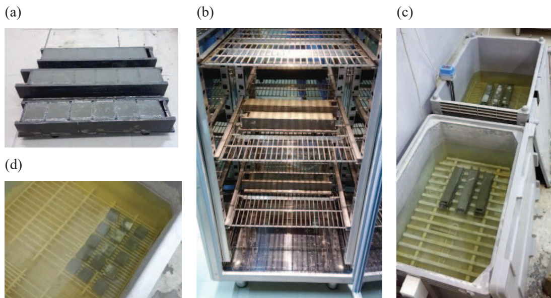
Rys. 4.8. (a) Zaformowane próbki zaprawy, (b) Próbki umieszczone w chłodziarce w temperaturze 9 °C, (c) Próbki pielęgnowane w temperaturze 24 °C i 40 °C, (d) Rozformowane próbki w kąpeli wodnej
