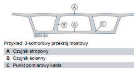
Rys. 3.18. Przykładowy układ czujników pomiarowych [164]
