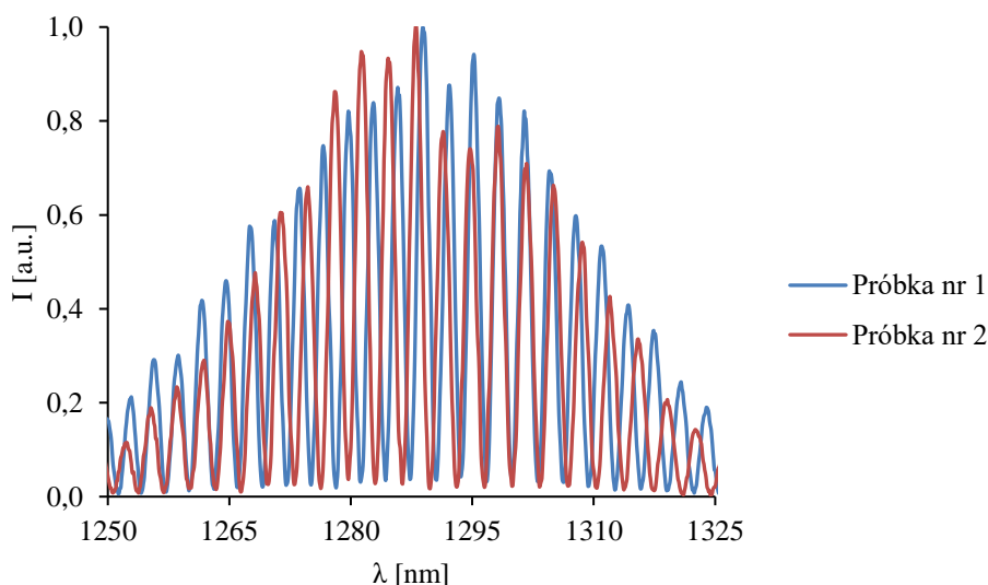
Rys. 4.1.5. Przykładowe interferogramy zarejestrowane w trakcie pomiarów dwóch próbek krwi o różnych parametrach hematologicznych.
