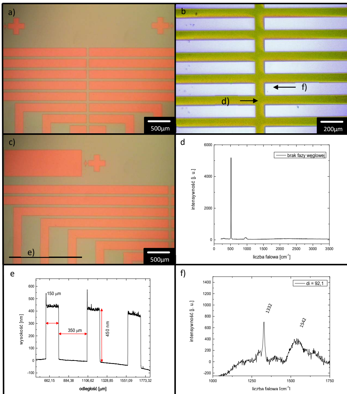
Rys. 49 Poziom izolacji wykonany w procesie „01” a,b,c) zdjęcia mikroskopowe w różnych powiększeniach, d) Spektroskopia Ramana wykonana na obszarze trawienia, e) rozmiary struktury zmierzone z użyciem profilometru (krzywizna podłoża wynikająca z zakresu pomiaru ok. 2cm i niedokładności pomiarowej urządzenia), f) pomiar Ramana dla obszaru diamentu po odcięciu linii bazowej i znalezieniu położenia pików.
