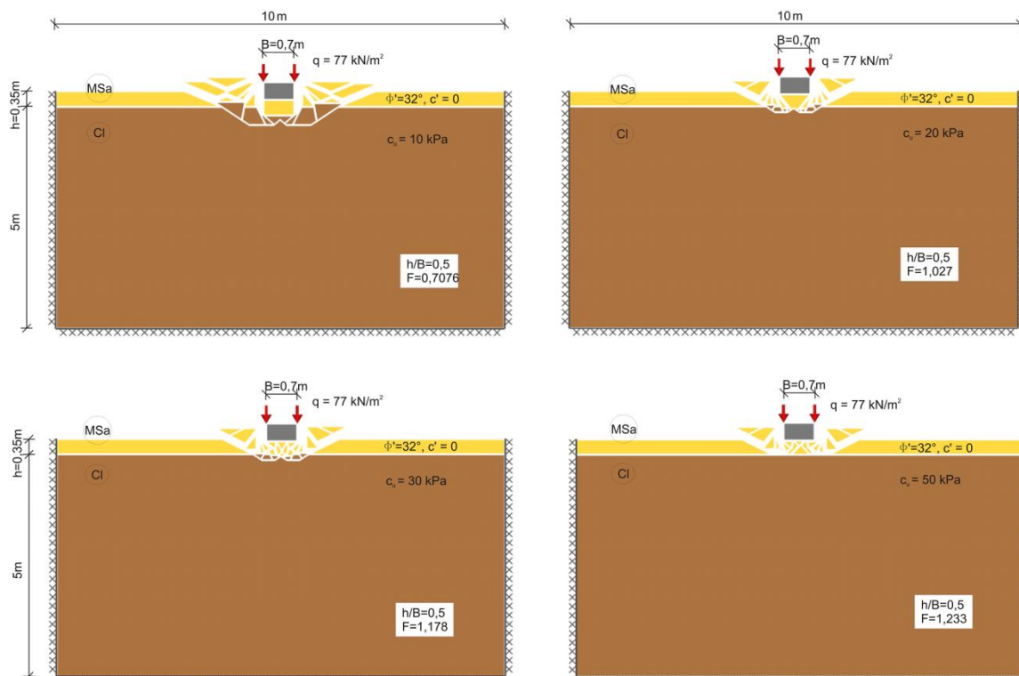
Rysunek B.19 Mechanizmy zniszczenia przy względnej miąższości platformy \left(\frac{h}{B}\right) = 0,5 i różnych wartościach wytrzymałości na ścinanie bez odplywu c_u (Eurokod 7, podejście 2b*)
