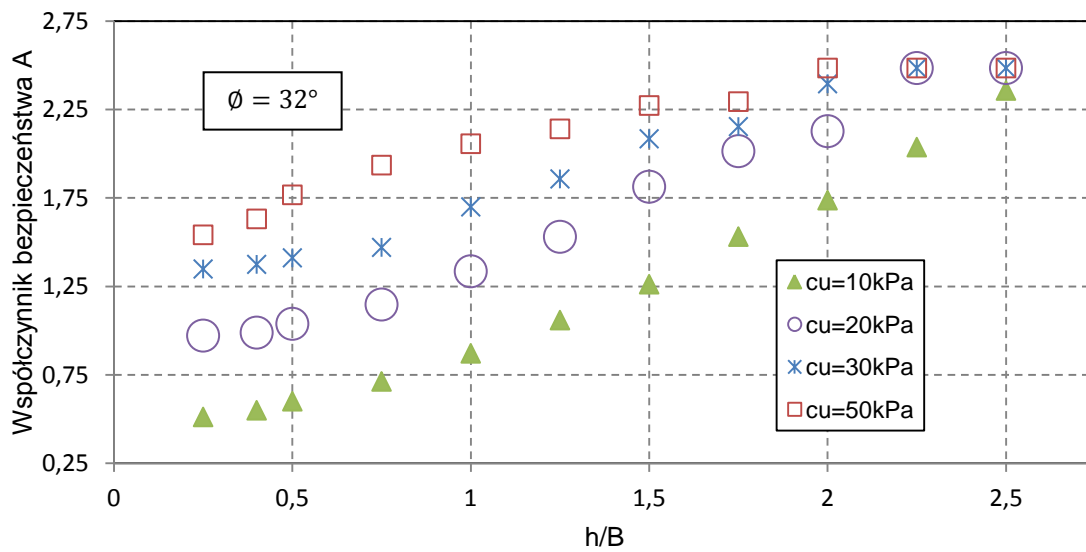
Rysunek A.36 Współczynnik bezpieczeństwa A w zależności od względnej mięszkości platformy roboczej ( \frac{h}{B} ) dla różnych wartości wytrzymałości na ścinanie bez odpływu c_u , \phi = 32^\circ .
