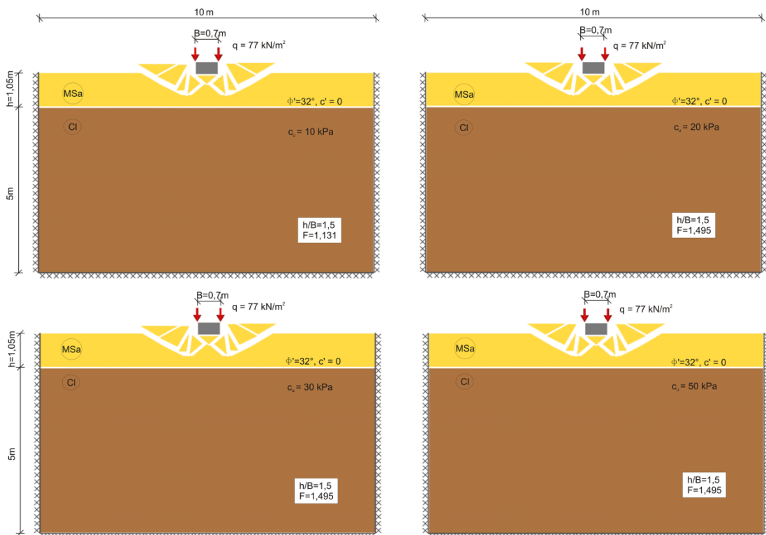
Rysunek A.5 Mechanizmy zniszczenia przy względnej miąższości platformy (\frac{h}{B}) = 1,5 i różnych wartości wytrzymałości na ścinanie bez odpływu c_u (Eurokod 7, podejście 1b)
