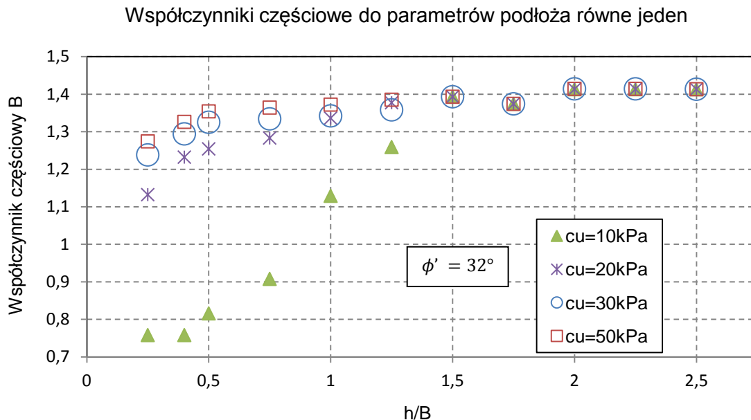
Rysunek 5.32 Współczynnik częściowy B w zależności od względnej miąższości platformy roboczej \left(\frac{h}{B}\right) dla różnych wartości wytrzymałości na ścinanie bez odplywu c_u (współczynniki częściowe do parametrów geotechnicznych podłoża równe jeden).
