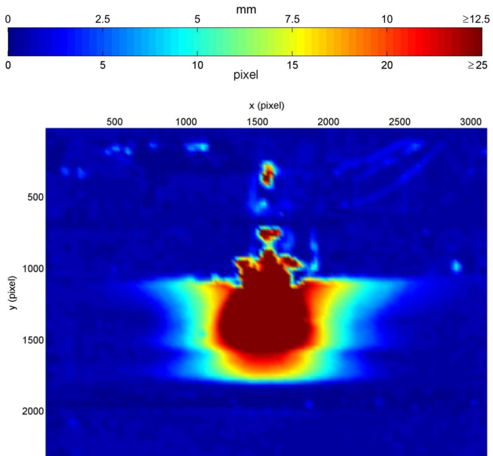
Rysunek 6.28 Pola przemieszczeń PIV układ 50 cm pianki i 10 cm piasku bez geosyntetyku, badanie nr 2, (s/B) = 0,1
