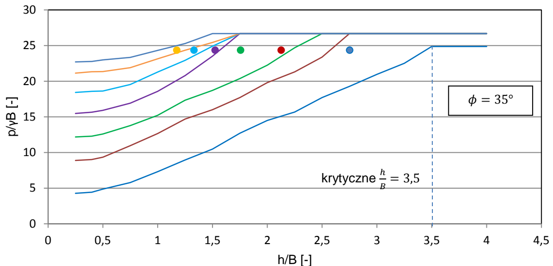
Rysunek 5.41 Przykładowy wykres pomocniczy do określenia krytycznej wartości względnej miąższości platformy ( \frac{h}{B} ) Michałowski i inni, 1995
