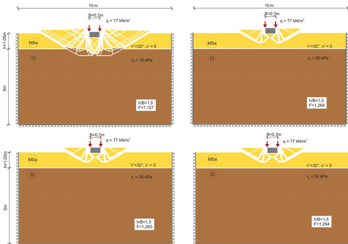
Rysunek B.20 Mechanizmy zniszczenia przy względnej miąższości platformy \left(\frac{h}{B}\right) = 1,5 i różnych wartościach wytrzymałości na ścinanie bez odplywu c_u (Eurokod 7, podejście 2b*)
