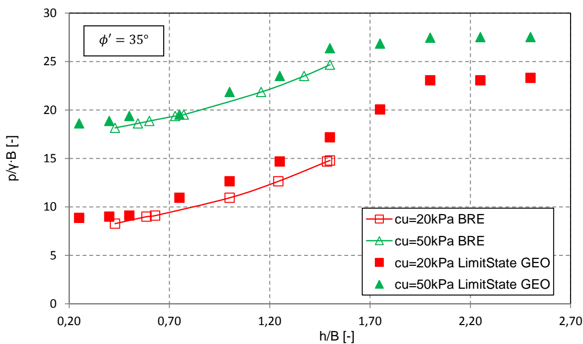
Rysunek 5.36 Znormalizowana nośność podłoża według podejścia BRE 470 oraz programu LimitStateGEO przy użyciu współczynników częściowych równych jeden, kąt tarcia wewnętrznego \phi' = 35^\circ
