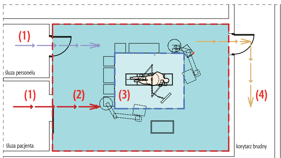
rzut sali operacyjnej z pokazaniem powiązań funkcjonalnych z sąsiednimi pomieszczeniami i różnych poziomów bezpieczeństwa
