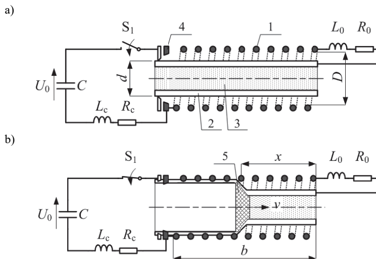
Rys. 1. Schemat ideowy działania generatora magnetokumulacyjnego: a) stan początkowy układu, b) kompresja pola magnetycznego wywołana procesem rozpęczenia twornika, 1 – uzwojenie generatora, 2 – twornik, 3 – materiał wybuchowy, 4 – łącznik (ang. crowbar), 5 – fala detonacyjna wywołana materiałem wybuchowym, C – bateria kondensatorów naładowana do napięcia U_0 , L_c , R_c – indukcyjność, rezystancja połączeń, L_0 , R_0 – indukcyjność i rezystancja cewki obciążenia, b – całkowita długość cewki generatora, x – efektywna długość cewki generatora w trakcie procesu generacji d – zewnętrzna średnica twornika, D – wewnętrzna średnica uzwojenia
