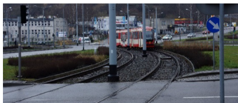
Rys. 5. Przykłady zagrożeń na sieci tramwajowej w Gdańsku
