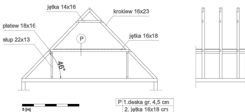
Rys. 5. Uproszczonego schematu więźby dachowej domu podcieniowego w Rybinie. (opracowanie autora)
