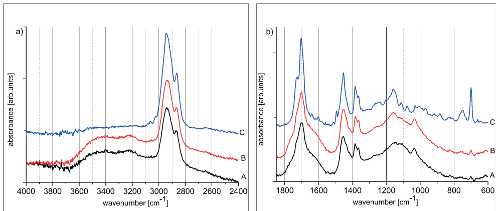
Abb. 3: Vergleich der FT-IR (ATR)-Spektrn von Geiseltal-Retinit (A, B) und Krantzit (C): a) 4000–2400 \text{cm}^{-1} und b) 1800–600 \text{cm}^{-1} .
