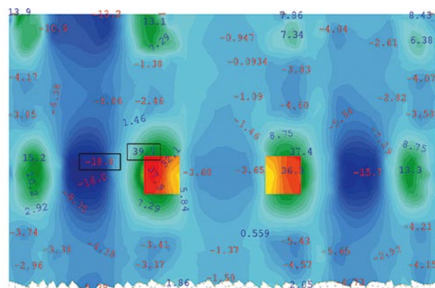
Rys. 15. Momenty zginające M_{xx} (kNm/m) dla fazy I
