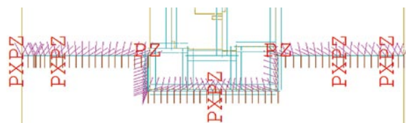
Rys. 2. Dylatacja konstrukcyjna
