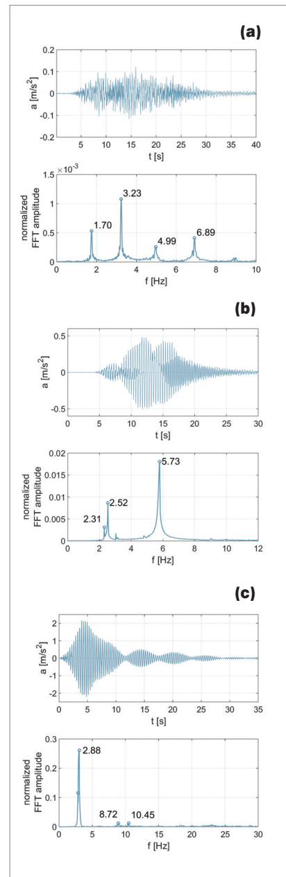
Rys. 9. Reprezentatywne przebiegi przyspieszeń wraz z odpowiadającymi im transformatami Fouriera dla kładki (a) nad drogą S8 w punkcie a5z od wymuszenia biegiem swobodnym grupy 12 osób (b) nad Trasą Uniwersytecką w Bydgoszczy w punkcie a1z od biegu synchronicznego grupy 9 osób (c) nad ulicą Chwarznieńską w Gdyni w punkcie a5z od wymuszenia marszem synchronicznym grupy 3 osób
