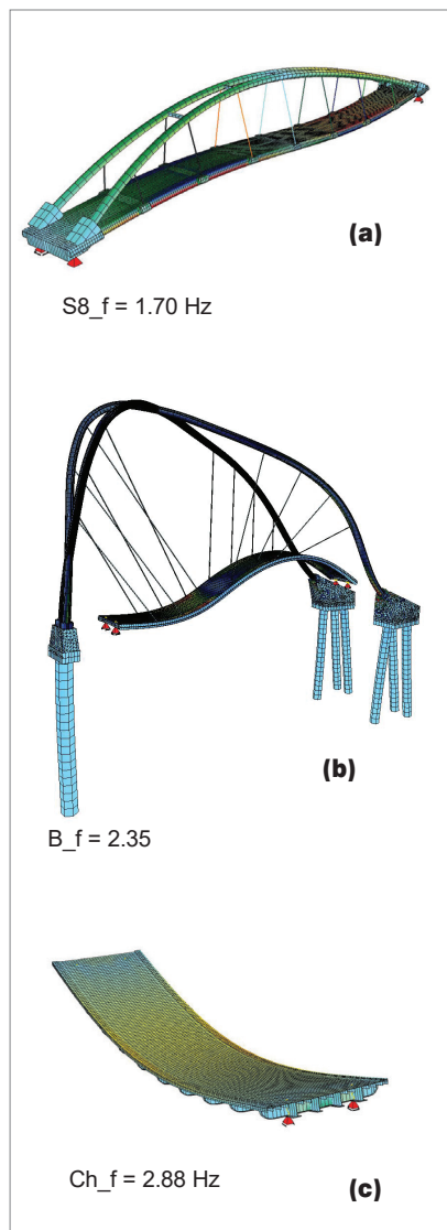
Rys. 6. Pierwsze giętne postaci drgań wraz z odpowiadającymi im częstotliwościami dla kładki (a) nad drogą S8 (b) nad Trasą Uniwersytecką w Bydgoszczy (c) nad ulicą Chwarznieńską w Gdyni
